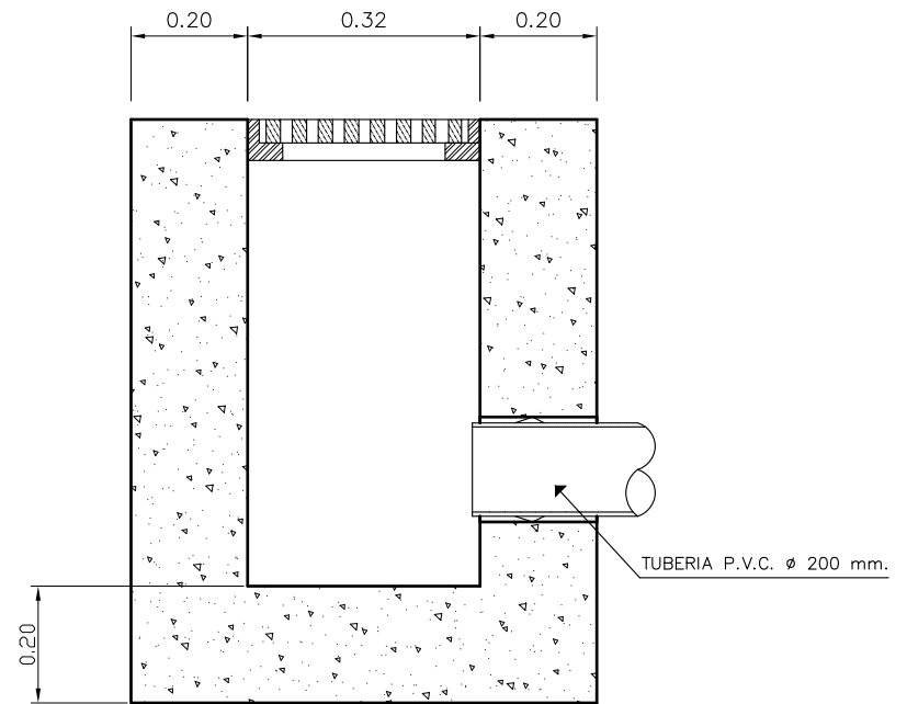
SECCION C-C
