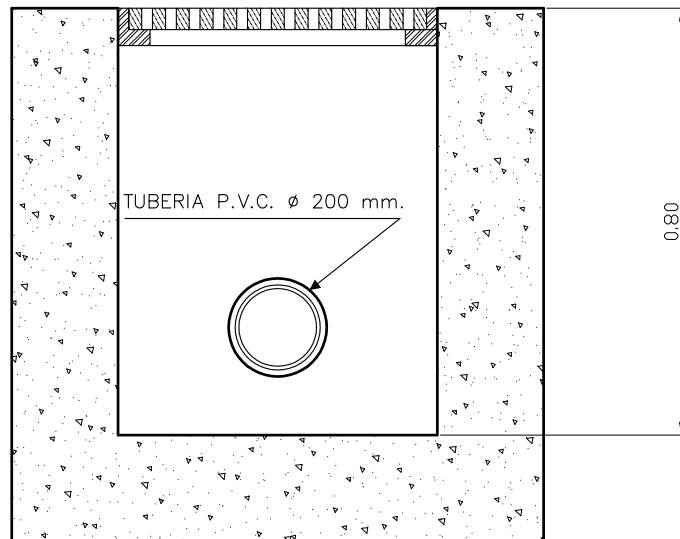
SECCION B-B
