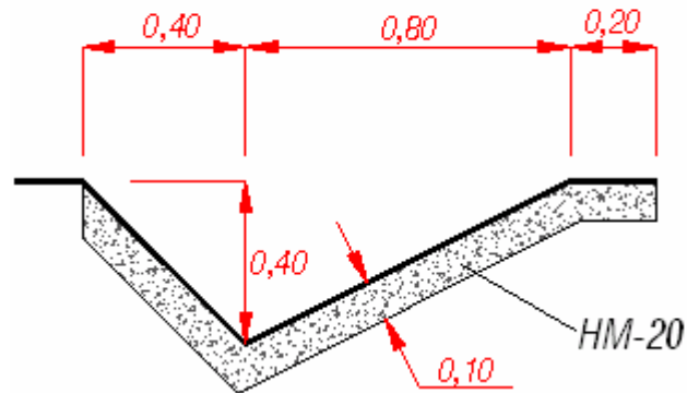
Cuneta revestida
